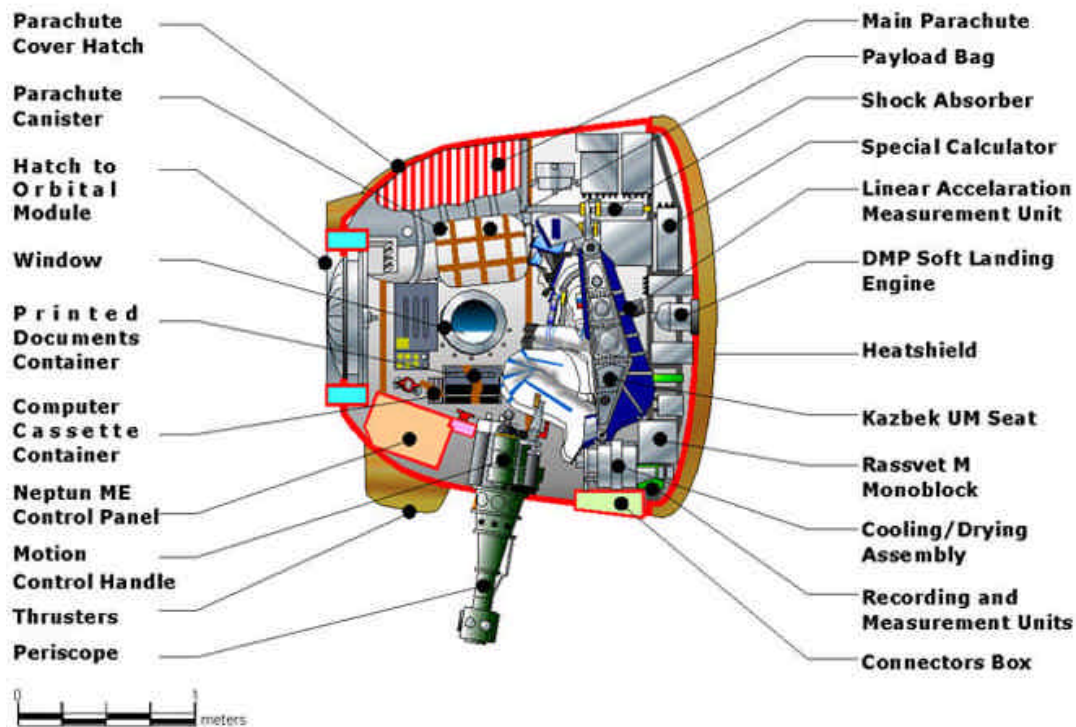
Soyuz TMA Landing or Command Module (Image: G. De Chiara Mars Center/2002)
